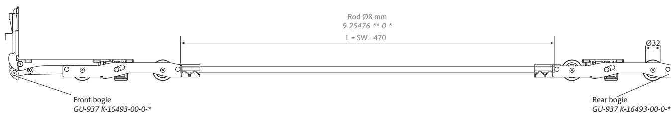
Fig.: L&S bogie GU-937
