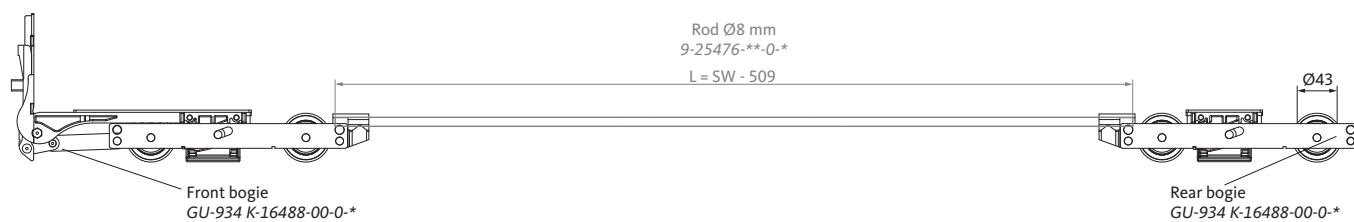
Fig.: L&S bogie GU-934
